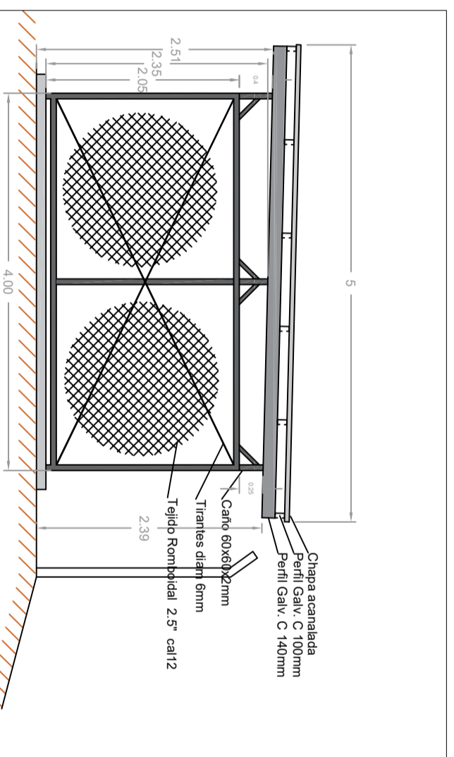
Cerramiento para boxes de residuos voluminosos - Lateral
